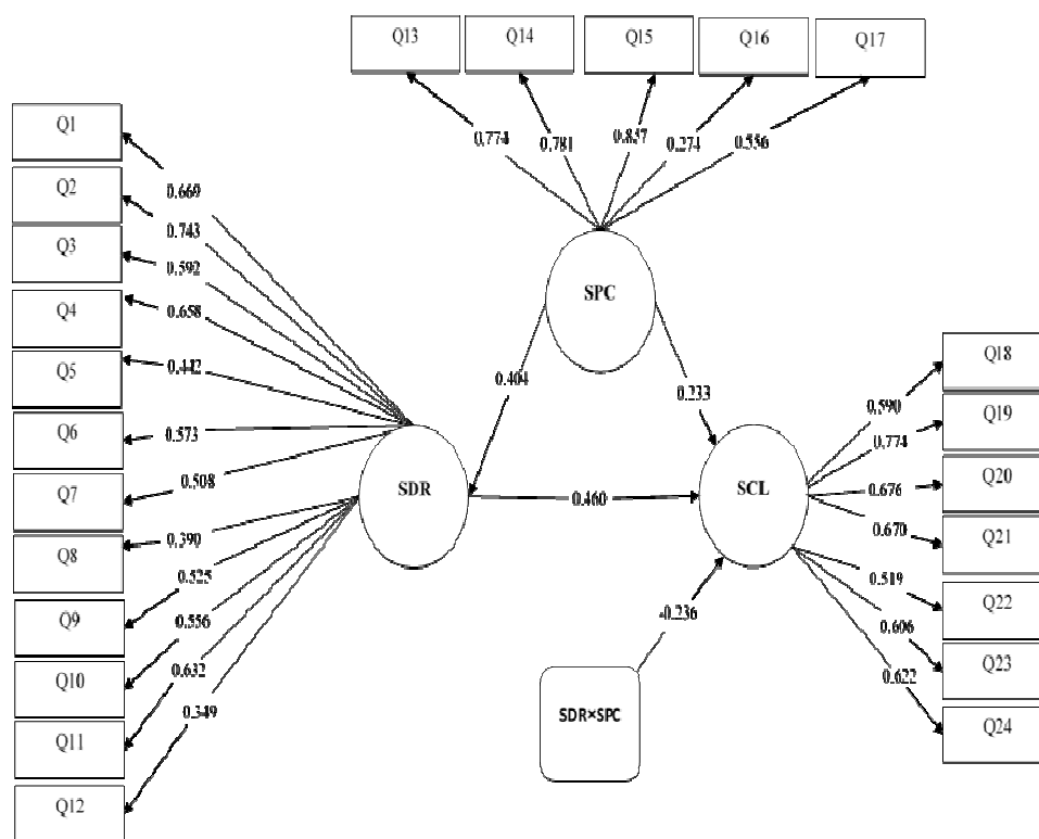
شکل ۳ مدل معادلات ساختاری در حالت ضرایب استاندارد
